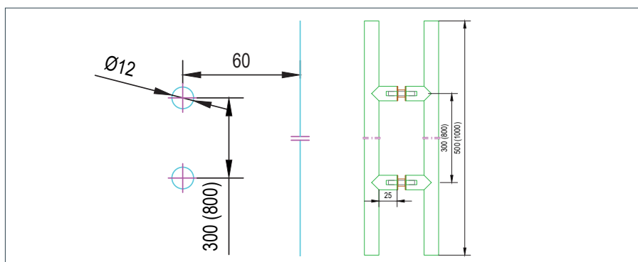
GM STANGENGRIFF (FÜR DEN INNENBEREICH)
