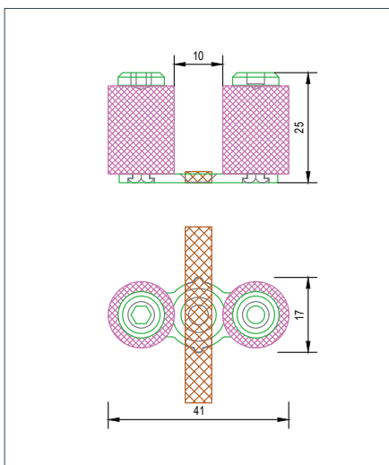
GM PIN MIT FILZ
