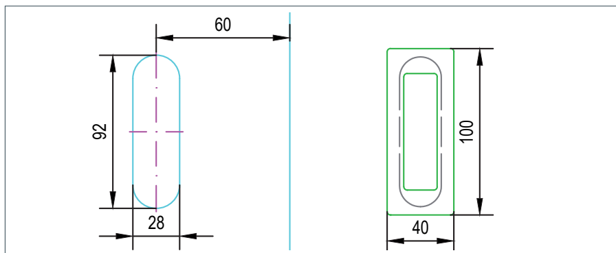
GM MUSCHELGRIFF (ECKIG)
