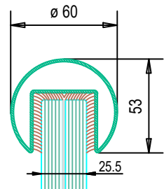
Solid 24 (Handlauf) Art.Nr.: 564060-00-80-000
