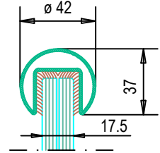
Solid 16 (Handlauf) Art.Nr. 564250-00-80-000
