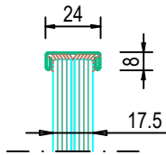
Extralight 16 (Kantenschutz) Art.Nr.: 564641-00-80-000
