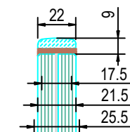
GM Glass Stripe (Kantenschutz) schwarzes Silikon Art.Nr. 520012-00-80-33 graues Silikon Art.Nr. 520013-00-80-034
