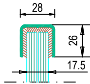
Light 16 (Handlauf) Art.Nr.: 564228-00-80-000
