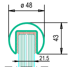
Solid 20 (Handlauf) Art.Nr.: 564048-00-80-000
