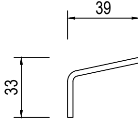
Abweiserverbinder Art.Nr: 516001-26-01-001
