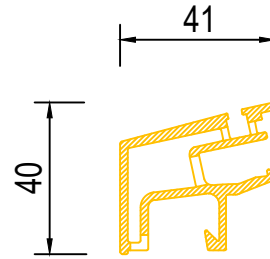
Abweiserprofil Art.Nr: 504197-01-01-001
