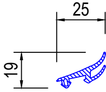
Silikonprofil Art.Nr: 534220-00-80-033
