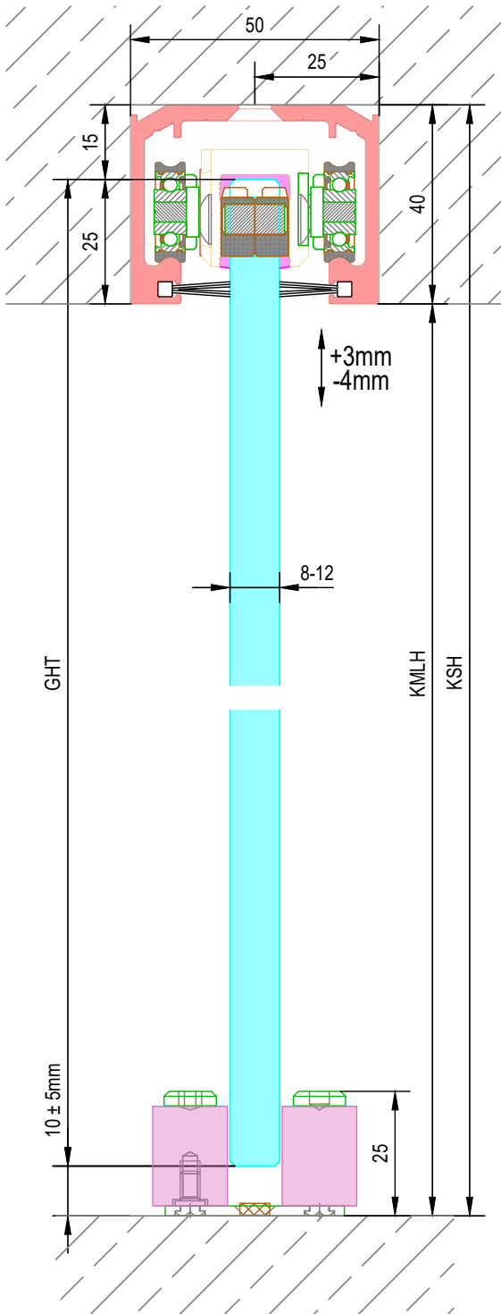
Flächenbündige Deckenmontage
