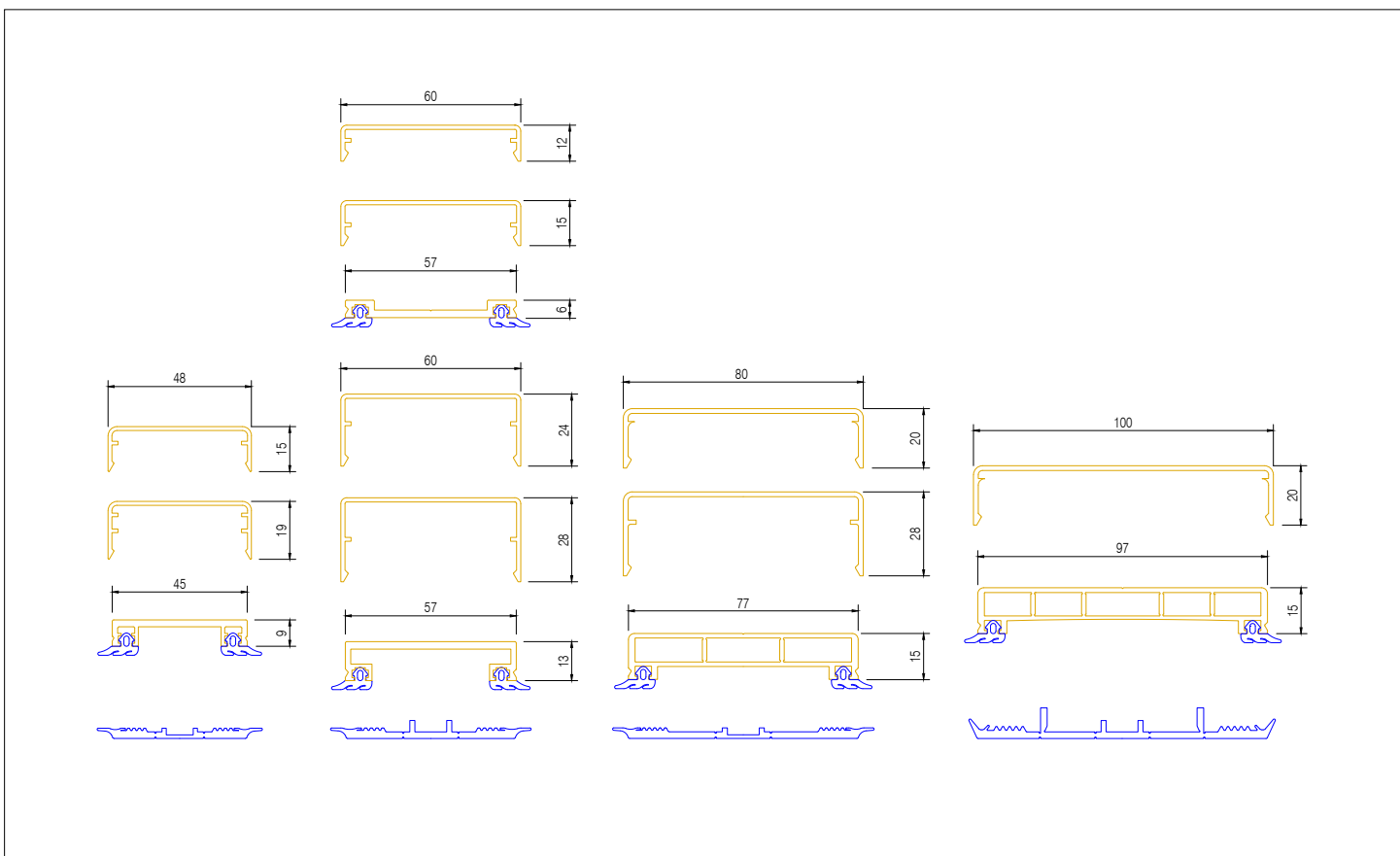
Klemprofile und dazugehörige Deckschalen in verschiedenen Größen erhältlich
