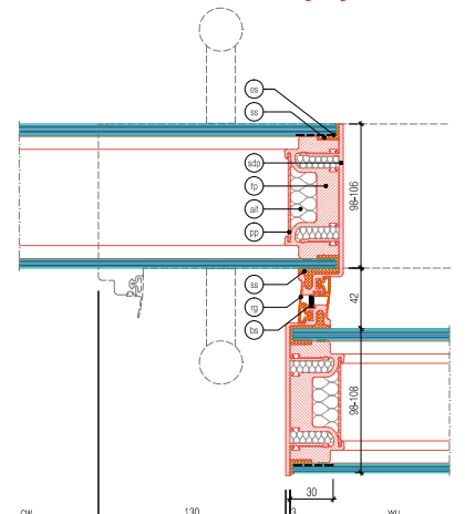
GM MARTITION® Plus Horizontalschnitt Schiebetür Griffgegensseite
