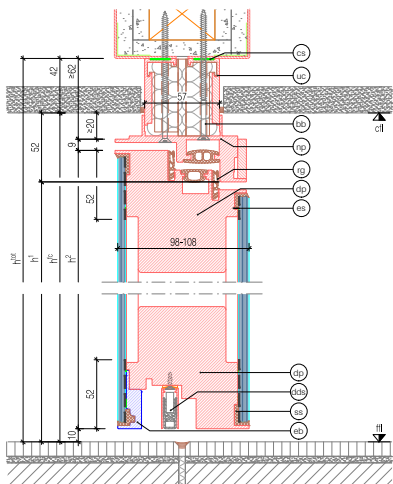
GM MARTITION® Plus Vertikalschnitt Drehtür
