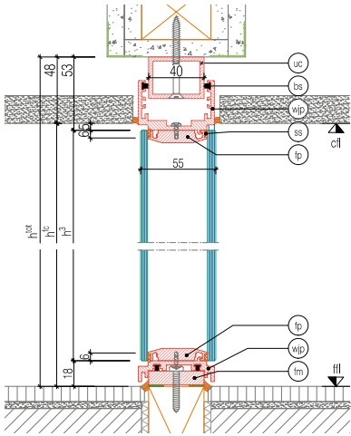
GM MARTITION® Light Vertikalschnitt Fixteil
