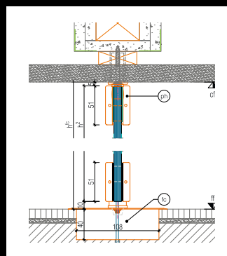
GM MARTITION® Mono Drehtür
