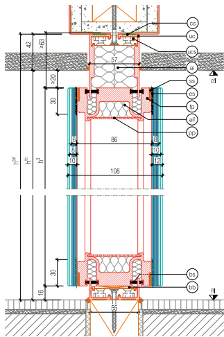
GM MARTITION® Plus Vertikalschnitt Wandteil
