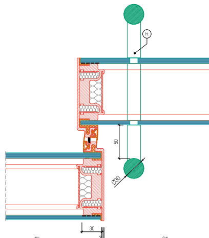
GM MARTITION® Plus Horizontalschnitt Schiebetür Griffseite
