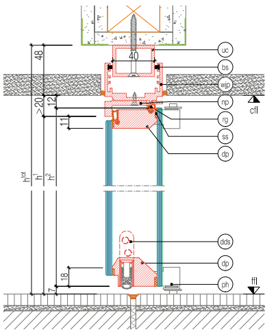
GM MARTITION® Light Vertikalschnitt Drehtür
