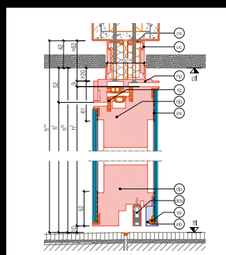
GM MARTITION® Plus Drehtür
