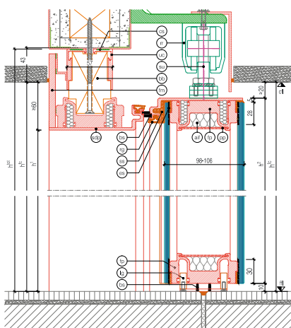
GM MARTITION® Plus Vertikalschnitt Schiebetür
