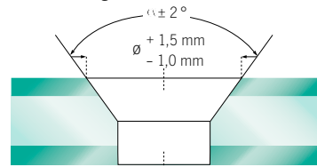
Senkbohrung
