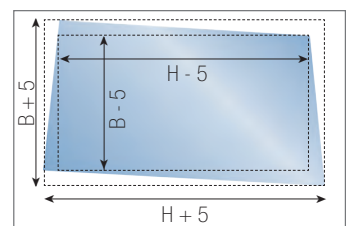
Abb. 4: Winkligkeit
