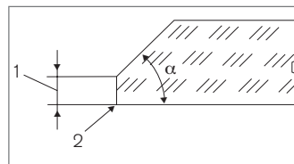
Abb. 5: Gehrungskante
