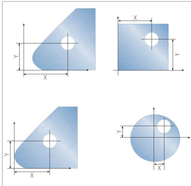
Abb. 13: Bohrlochlage
