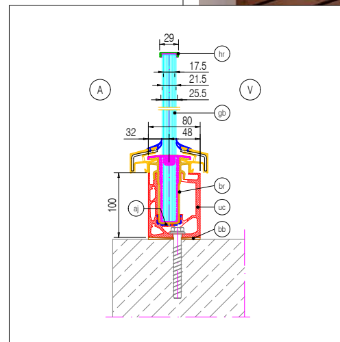
Zweite Dichtebene
