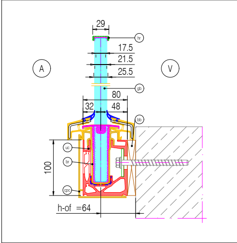
Zweite Dichteebene
