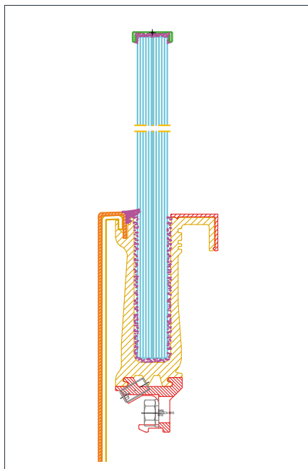
bauseitige Abdeckprofile: 0,6–3 mm Stoßkantenblech: 0,3–3,5 mm
