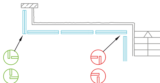
Geländerverlauf – Grundriss
